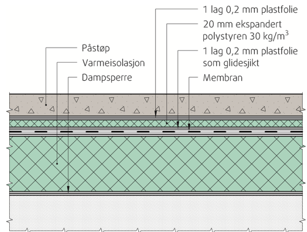
Fig.3 Eksempel på bruk av Mataki UnoTech FR som innebygget membran
